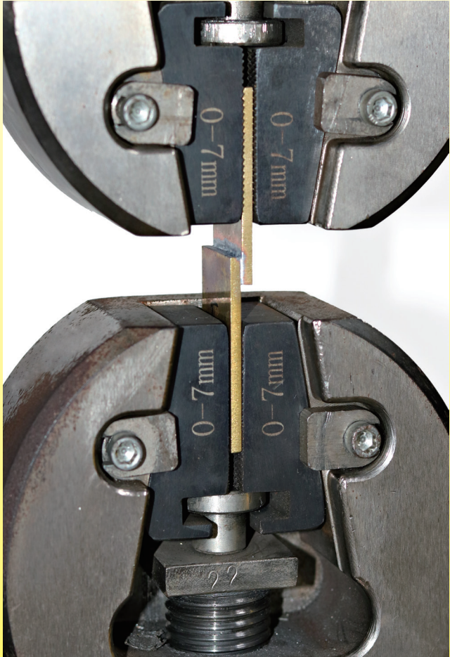
Especímenes probados según la resistencia a la tracción última de la soldadura. Valores medidos en nuestro propio equipo de pruebas a una velocidad de 0,05 mm/min
