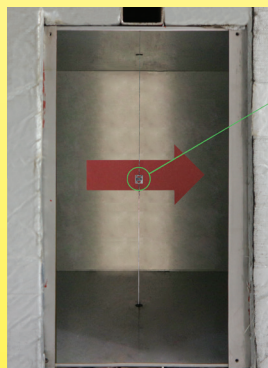
Posición de los enlaces térmicos o mecanismos de bulbo térmico en la corriente de aire para la medición del límite de temperatura umbral
