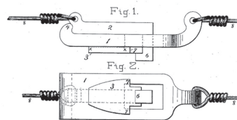
1890 Enlace fusible desmultiplicado ensamblado en un cable (patente de Frederick Grinnel N.º 432403)
